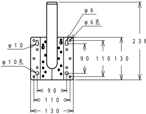
壁面取付寸法
