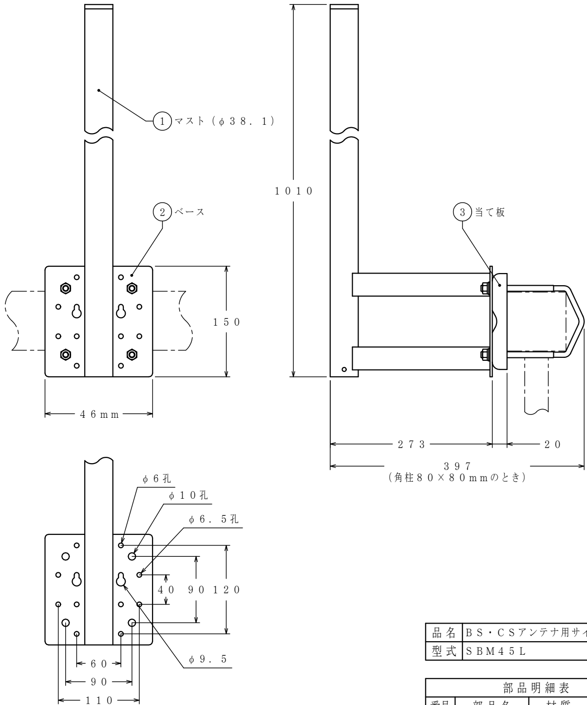
取付孔寸法図
