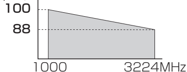
入力レベル (dB \mu V) 逆チルト入力の場合
