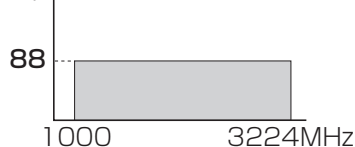
入力レベル (dB \mu V) フラット入力の場合
